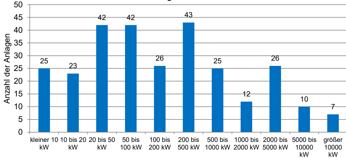
elektrische Leistung der WKA in Großstädten
