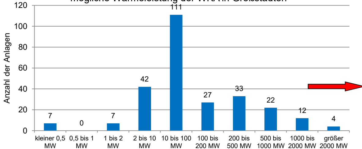
mögliche Wärmeleistung der WKA in Großstädten
