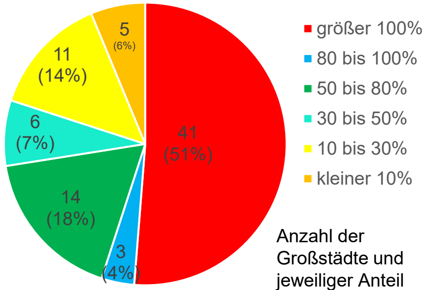
Fließgewässerwärmepotenzial bezogen auf den gesamten Raumwärmebedarf
